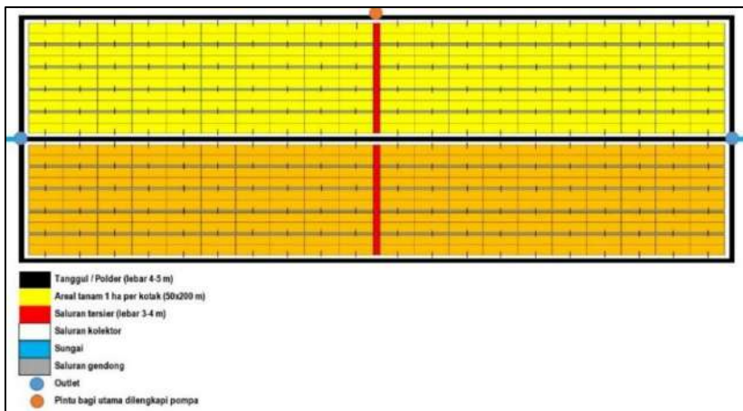
Gambar 4 Skema jaringan irigasi lahan rawa lebak berbasis mini polder
